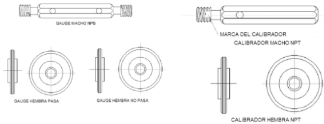
Figura 3.- Ejemplo de calibrador maestro macho o hembra
